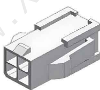
Molex 母壳 39-01-2041(4pin) 长23.9×宽11.6×高18mm
