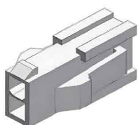
Molex 母壳 3901-2026(2pin) 长23.9×宽13.8×高11.6mm
