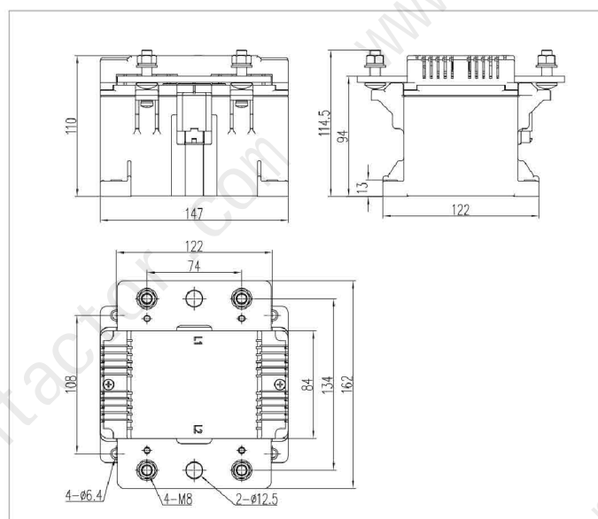
尺寸图&接线原理图 Dimension & Wiring
