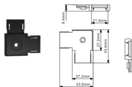
Corner module
