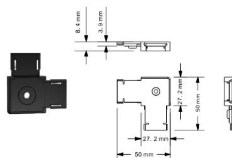
Corner module
