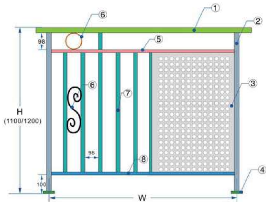
铝合金阳台护栏构造说明：
