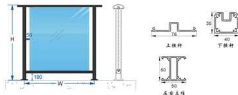
型号/Model: B-HYb-3
