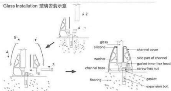
Glass Installation 玻璃安装示意
