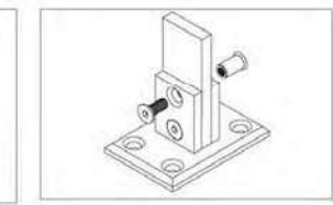
Balustrade bracket 侧板底板 MODEL: SJ-H195 Φ: 38/42.4/50.8
