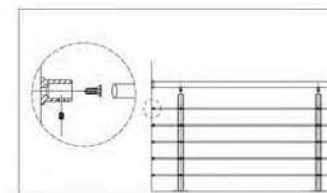
Wall flange 装墙法兰 MODEL: SJ-H157 Φ: 18/10/12/14
