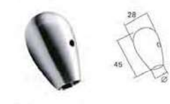
End cap 封头 MODEL: SJ-H158 Φ: 8/10/12
