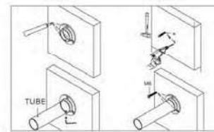
Balustrade bracket 侧板底板 MODEL: SJ-H194 Φ: 38/42.4/50.8
