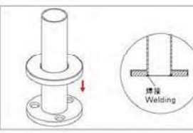
Balustrade bracket 侧板底板 MODEL: SJ-H196 Φ: 38/42.4/50.8
