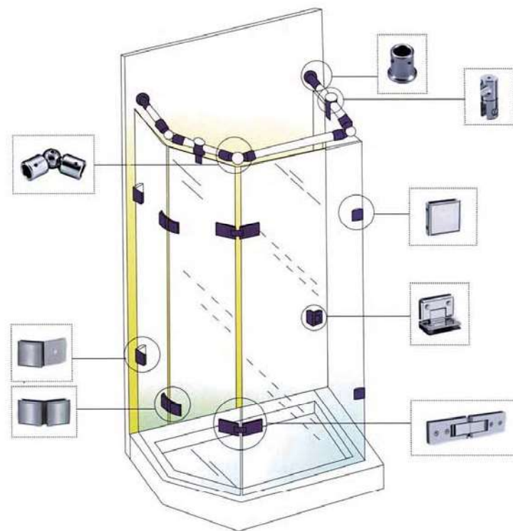
Shower room decomposition map 淋浴房分解图
