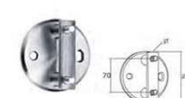
Balustrade bracket 侧板底板 MODEL: SJ-H196 Φ: 38/42.4/50.8
